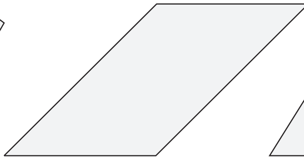
Parallelogramm
