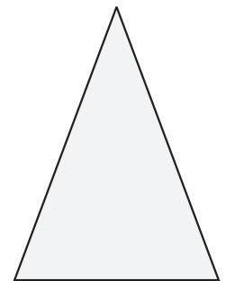
gleichschenkliges Dreieck
