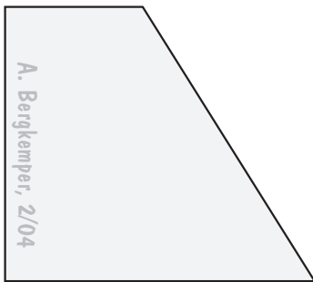
rechtwinkliges Trapez
