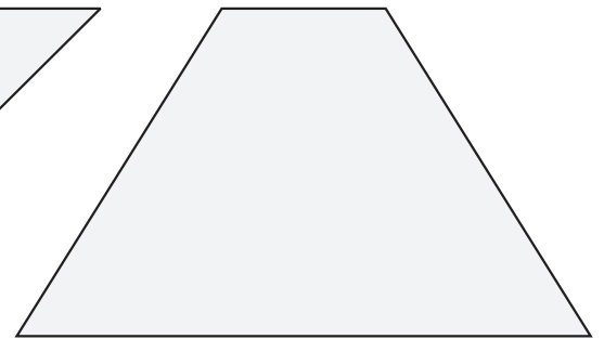
gleichschenkliges Trapez
