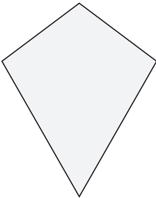
Drachenviereck
