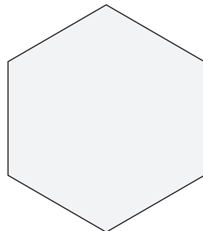
regelmäßiges Sechseck
