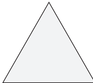
gleichseitiges Dreieck
