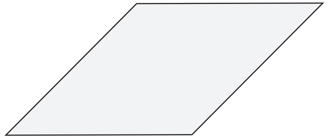
Raute
