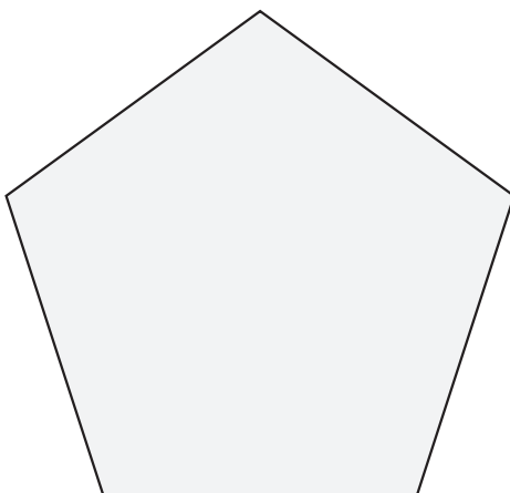
regelmäßiges Fünfeck
